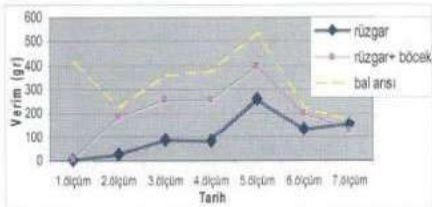
Şekil 7. Tozlaşma faktörlerinin ölçüm tarihlerindeki verim grafikleri
