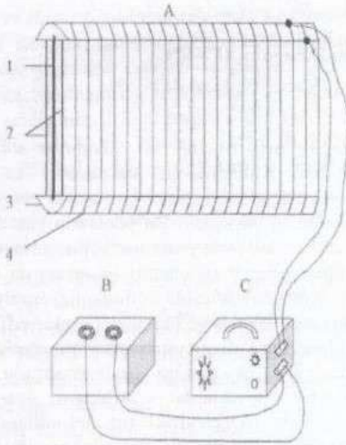
Şekil:1 Arı zehirinin toplanmasında kullanılan alet
